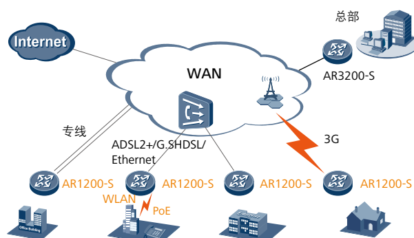
图 1. 广域互联场景
