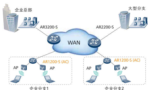
图 3. 无线AC管理场景
