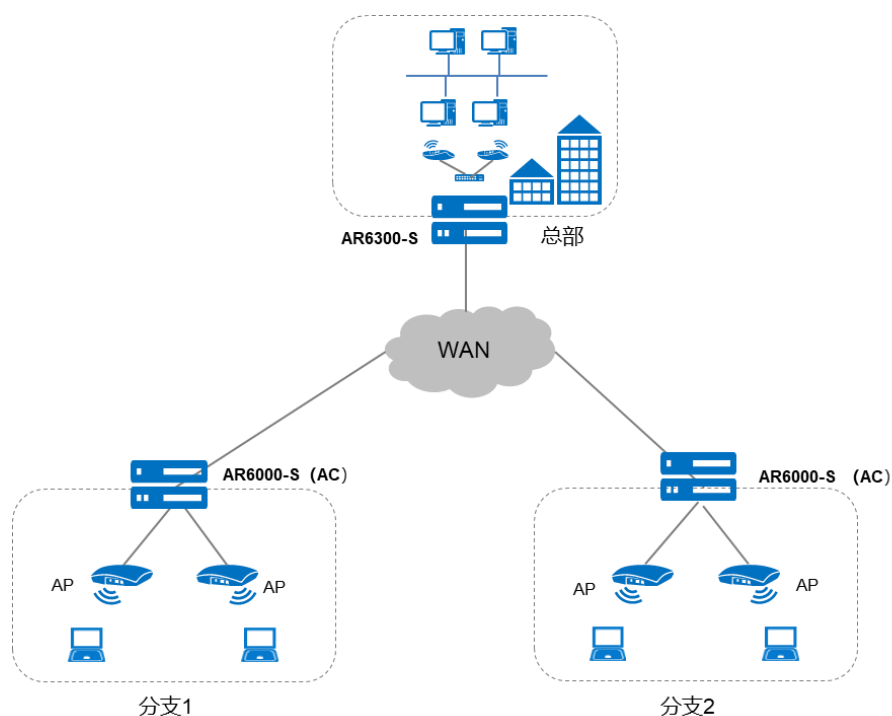
广域互联及无线接入场景组网图
